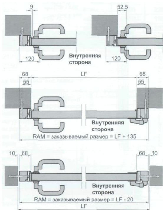
Профиль типа 1 (узкий профиль)
