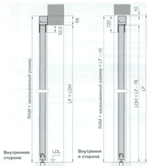
Монтаж двери сзади дверного проема
